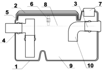
Принципова схема жириуловлювача серії СЖ "Оптима"
