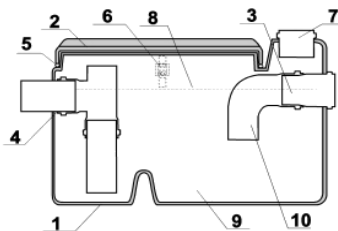
Принципова схема жиरोуловлювача серії СЖ "Оптима"
