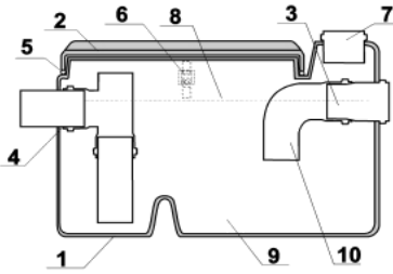
Принципова схема жируюловлювача серії СЖ "Оптіма"
